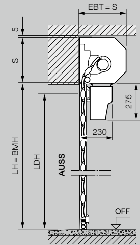
Campo de medidas para la puerta enrollable interior y exterior
